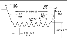
DETAIL C SCALE: 3/4
